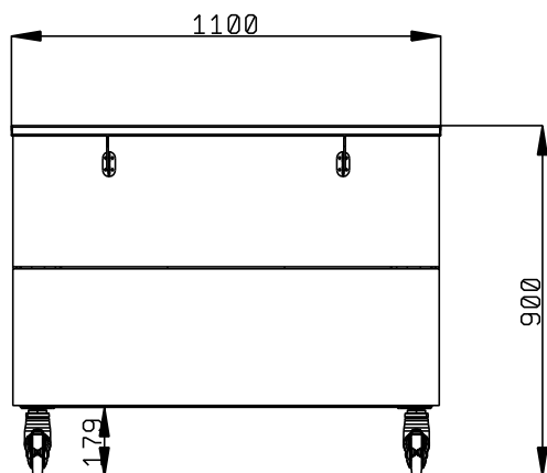
Alzado
